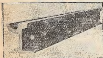
Rail à ornière type S.E.I.
